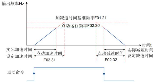
图 5-21 点动运行示意图
