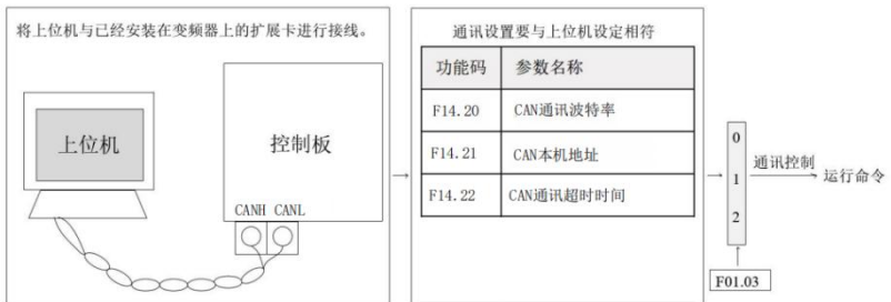
图 5-6 使用通讯设定运行命令
