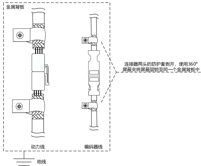
图 3-15 FD1X5 驱动器连接器侧动力线/编码器线屏蔽层 2*处理方式
