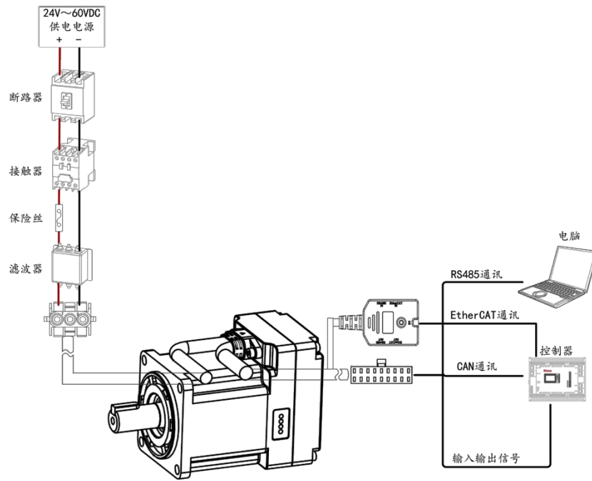
图 3-2 iSMK-AA/EA 系列集成电机外部连接方式
