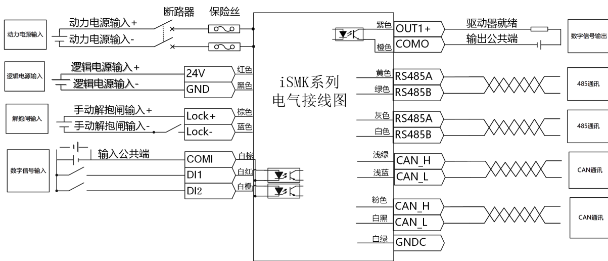
图 3-4 iSMK 系列电气接线图
