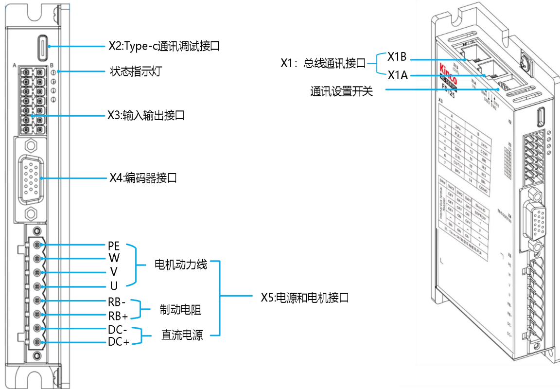
图 3-5 FD1X5 系列各部分名称
