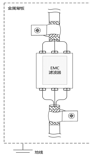
图 3-13 EMC 噪音滤波器安装示意图
