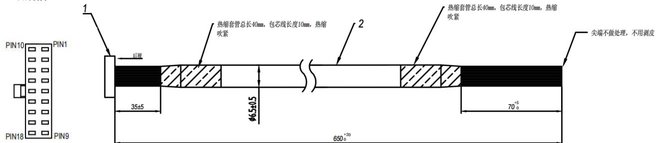
图 3-3 iSMK-AA 系列信号线缆外接端子
