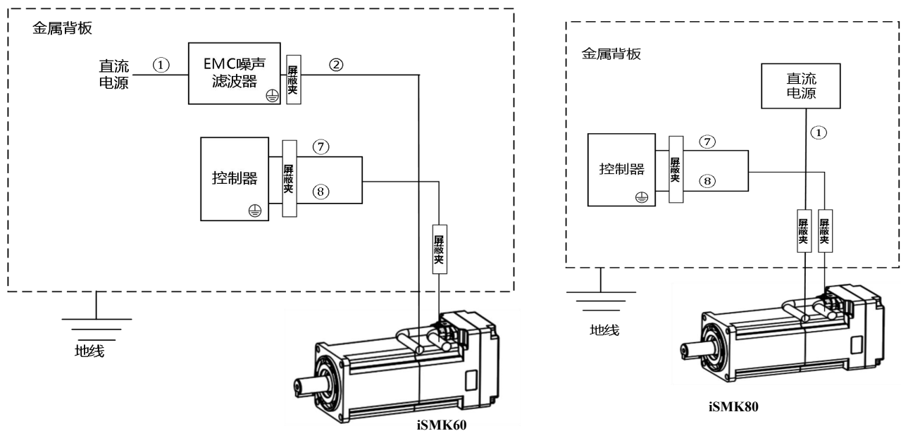
图 3-12 iSMK 系列驱动器安装环境示意图
