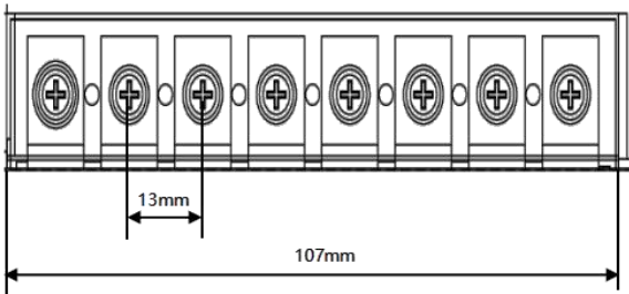
图 3-9 FD145 驱动器 X5 接口尺寸图
