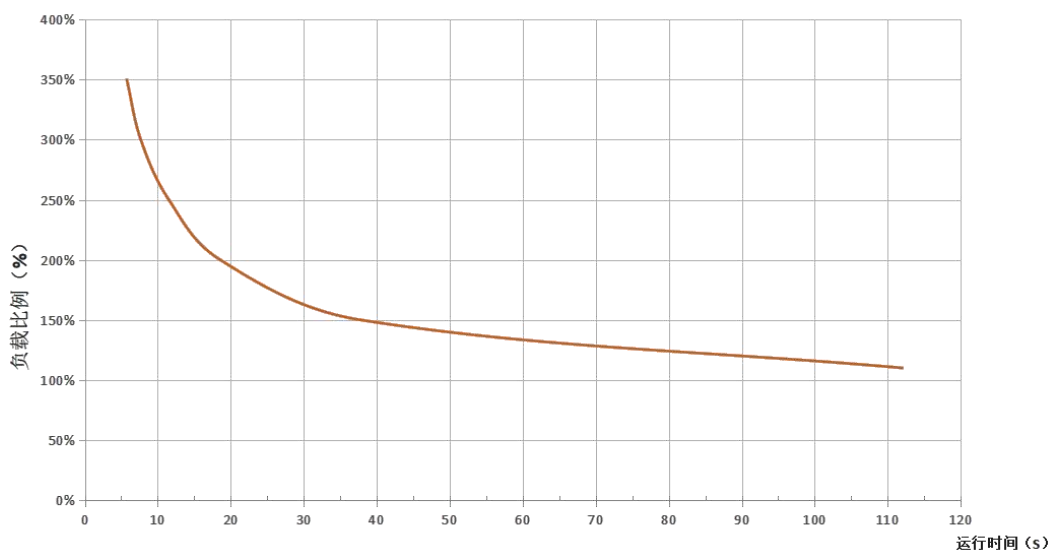
图 3-17 iSMK 过载特性曲线
