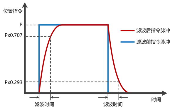
图 5 - 6 脉冲滤波说明
