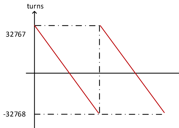
图 5-9 多圈数据范围
