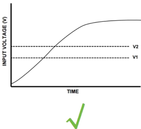
图 3-18 单调性电源
