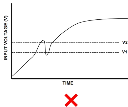
图 3-19 非单调性电源
