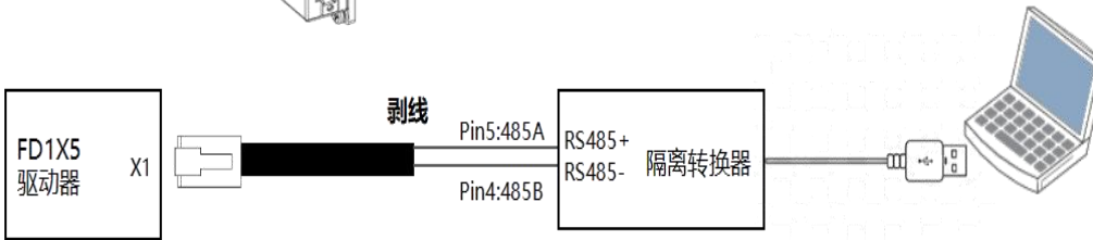
X1 接口通讯
