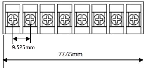
图 3-8 FD135 驱动器 X5 接口尺寸图
