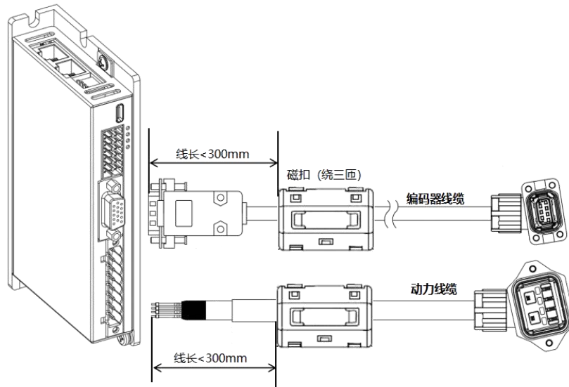
图 3-16 磁环安装图
