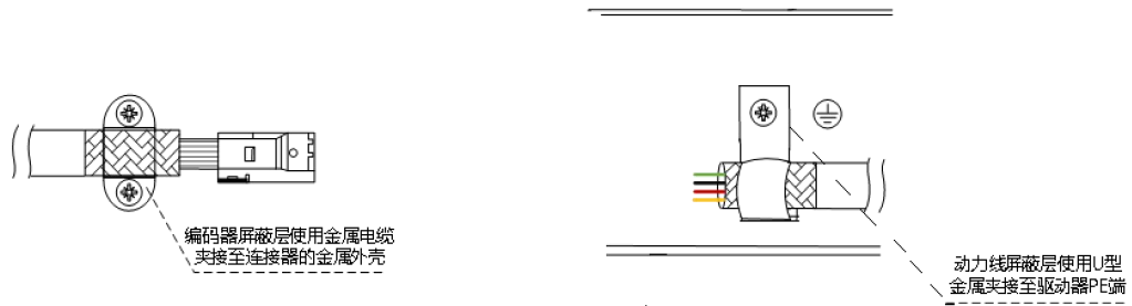
图 3-14 FD1X5 驱动器侧动力线/编码器线屏蔽层 1*处理方式
