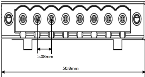
图 3-7 FD125 驱动器 X5 接口尺寸图
