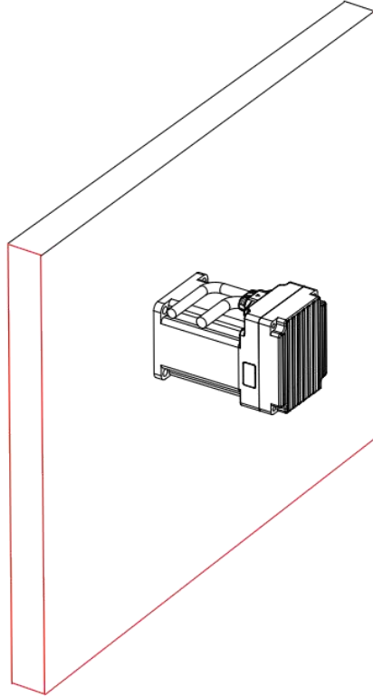
图 2-2 iSMK 辅助散热安装图
