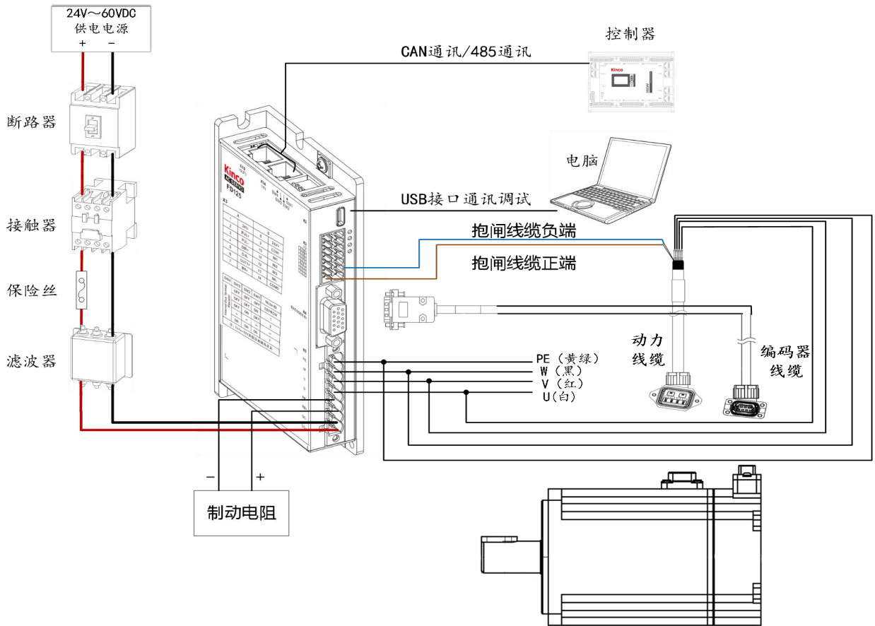
图 3-6 FD1X5 系列外部接线图
