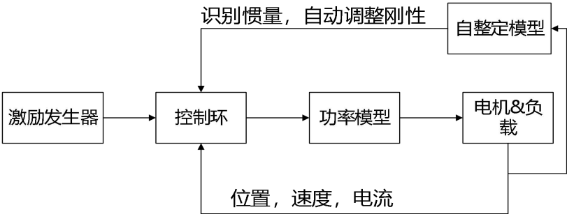
图 7-2 自整定框图
