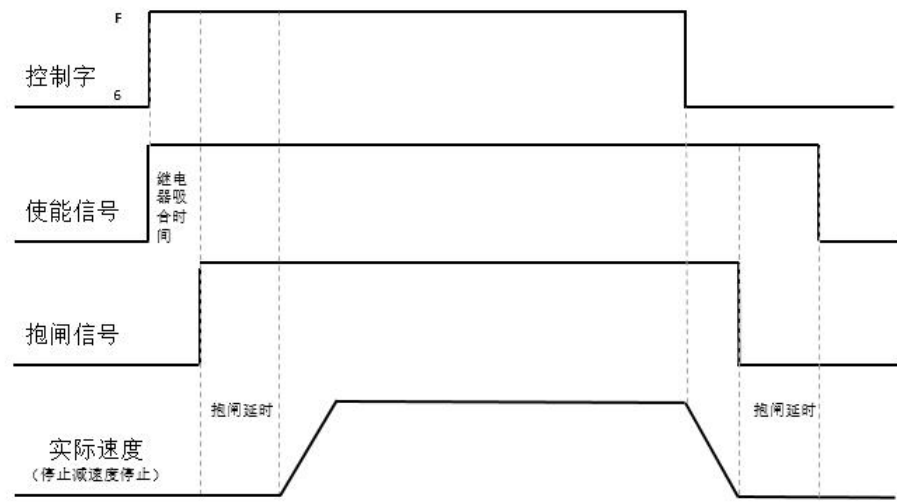
图 6-17 快速停止模式为 2 时电机抱闸时序
