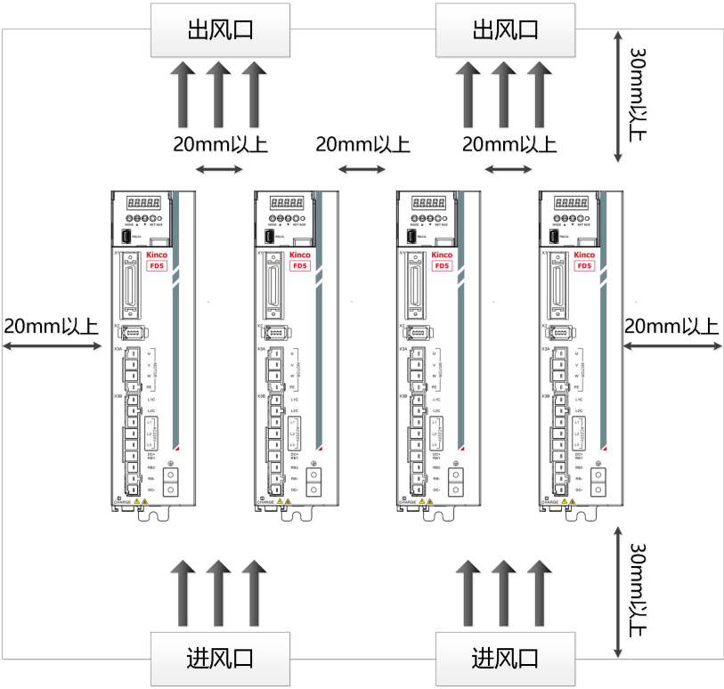
图 2-6 FD435/625 安装方向及要求
