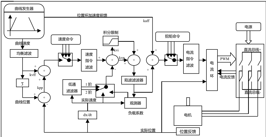
图 7-1 伺服系统控制结构框图
