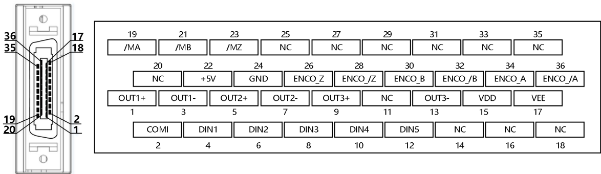
图 3-19 FD5-PA 驱动器外部输入输出端子引脚示意
