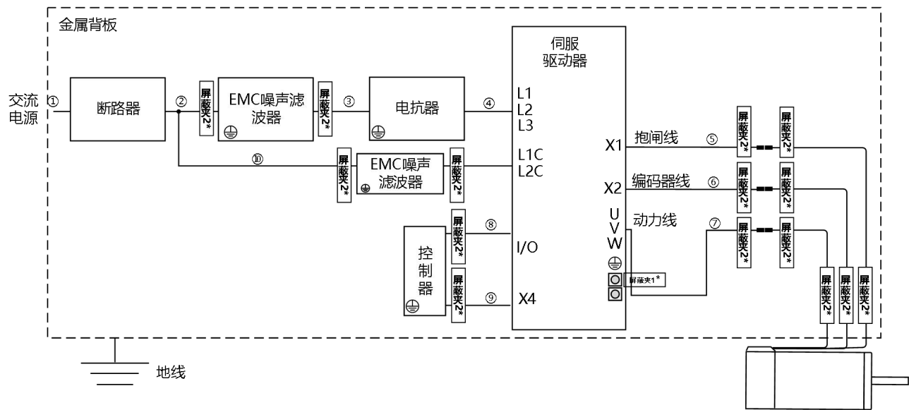
图 3-7 FD435/625 驱动器 EMC 设置条件示意图
