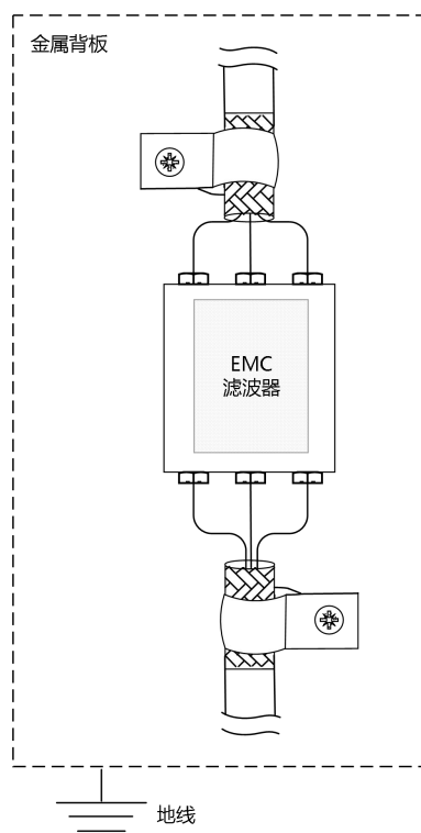
图 3-8 EMC 噪音滤波器安装示意图
