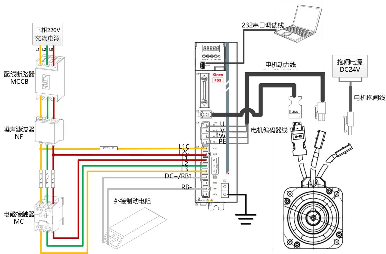
图 3-3 FD425 外部接线图
