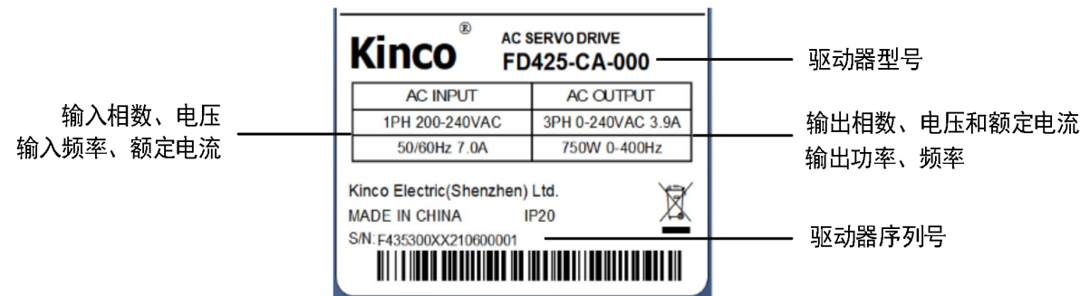
图 1-2 驱动器铭牌说明
