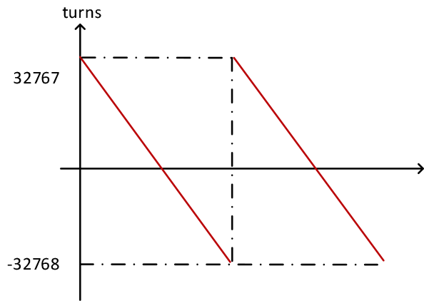
图 6-18 多圈数据范围
