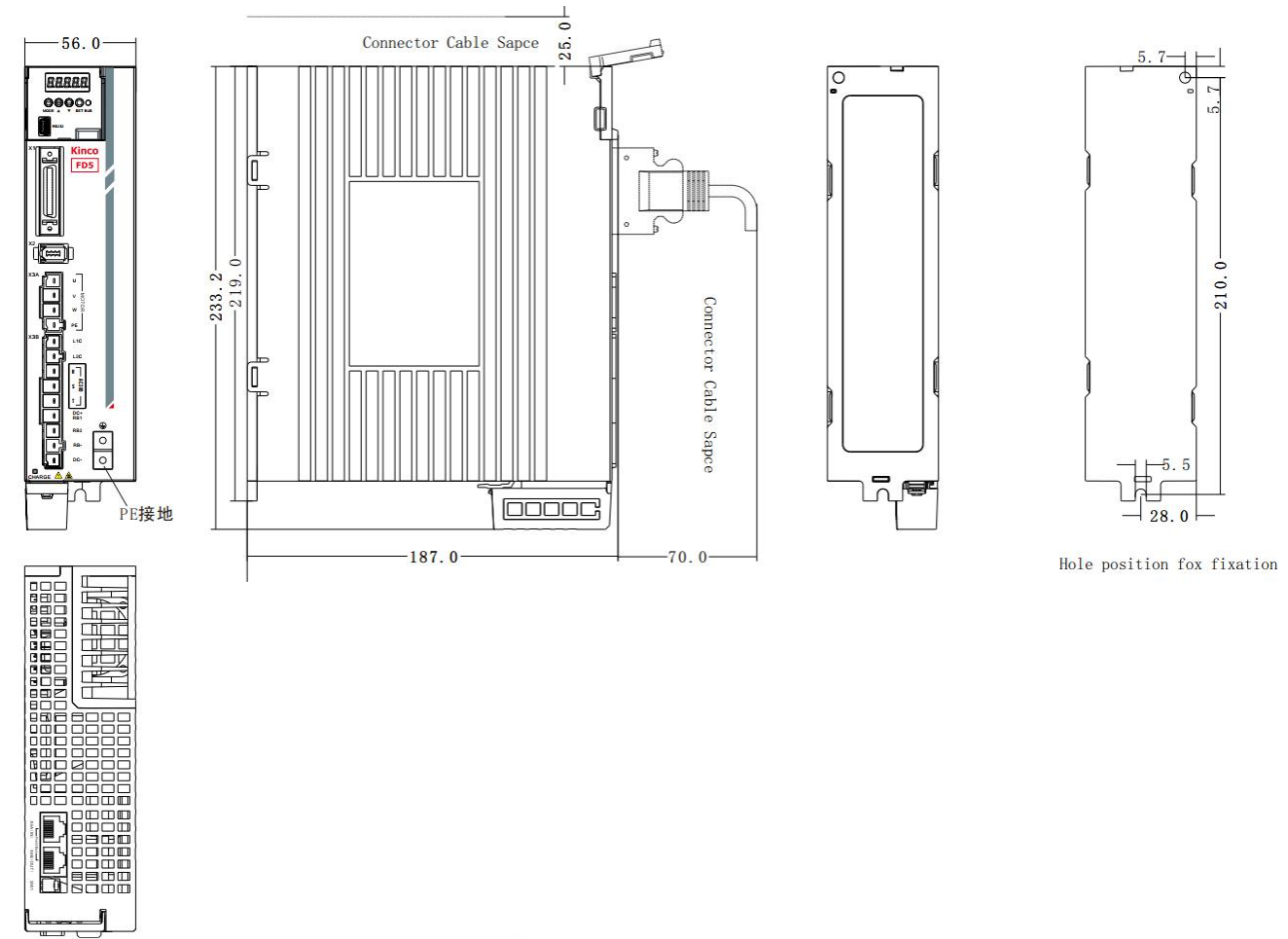
图 2-4 FD625-□A 产品安装图
