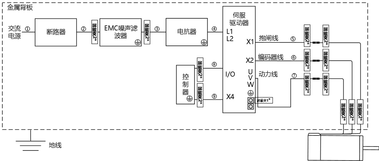
图 3-6 FD425 驱动器 EMC 设置条件示意图
