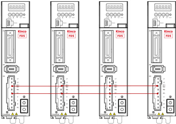
图 3-14 FD425 共直流母线
