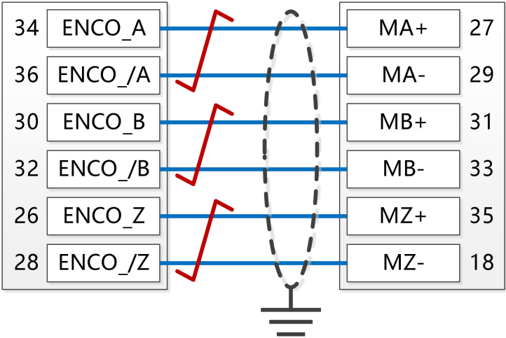
图 6-9 编码器线连接说明
