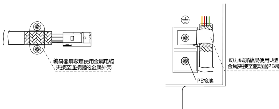
图 3-9 驱动器侧动力线/编码器线屏蔽层 1*处理方式
