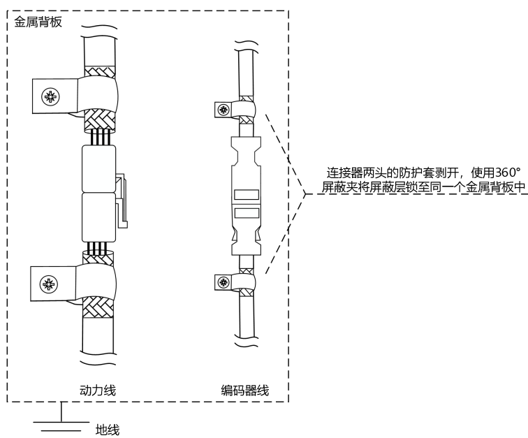
图 3-10 连接器侧动力线/编码器线屏蔽层 2*处理方式
