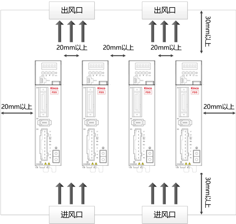
图 2-5 FD425 安装方向及要求
