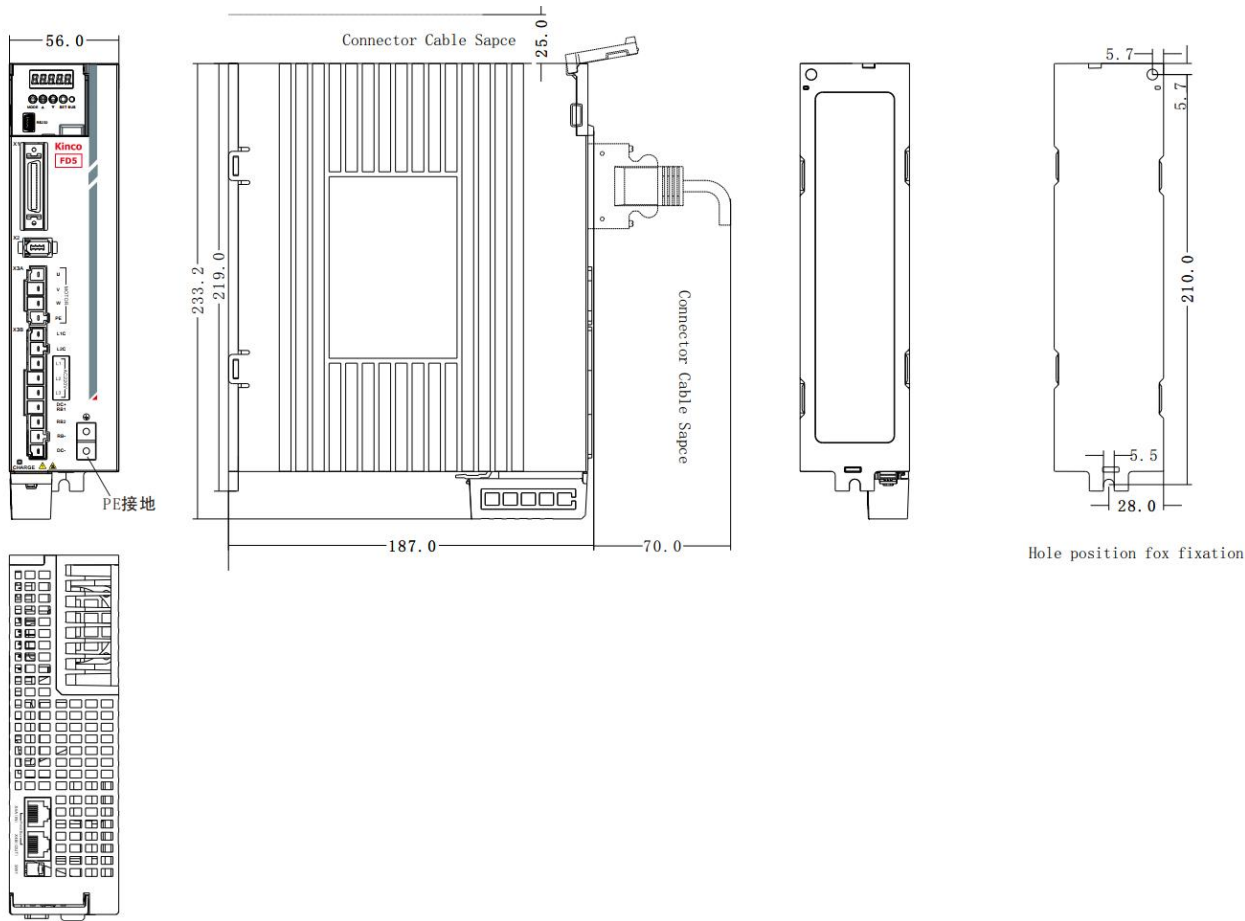
图 2-3 FD435-□A 产品安装图
