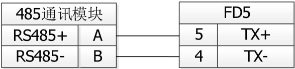
图 10-2 RS485 信号接线图
