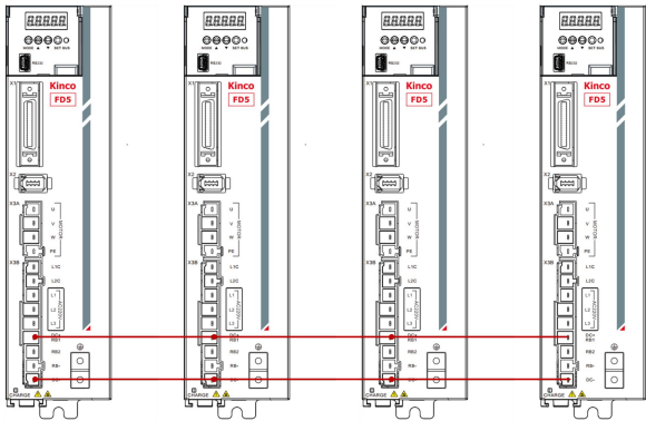
图 3-15 FD435/FD625 共直流母线
