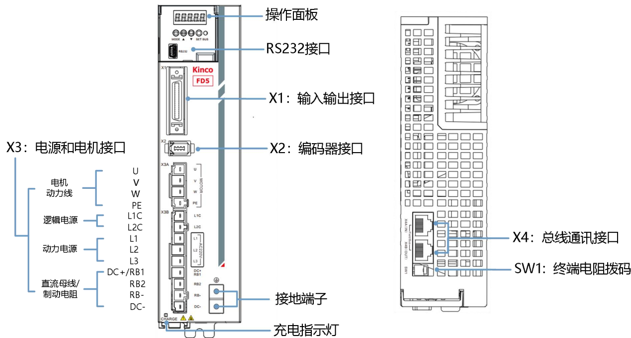
图 3-2 FD435/625 驱动器外观图
