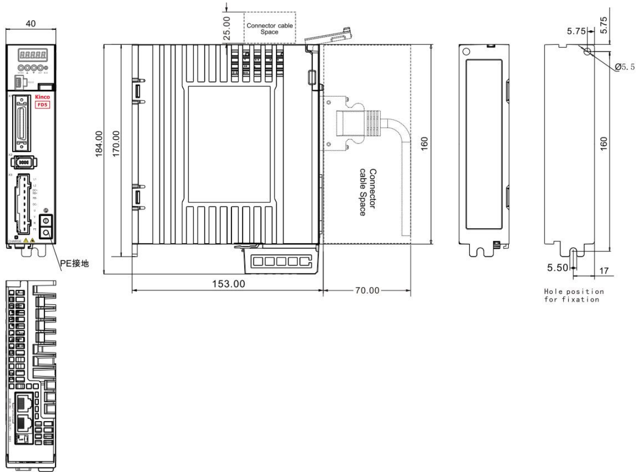
图 2-1 FD425-□A 产品安装图
