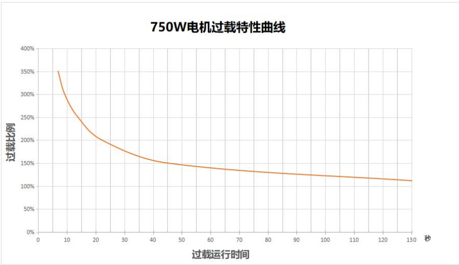
图 3-13 750W 电机过载特性曲线
