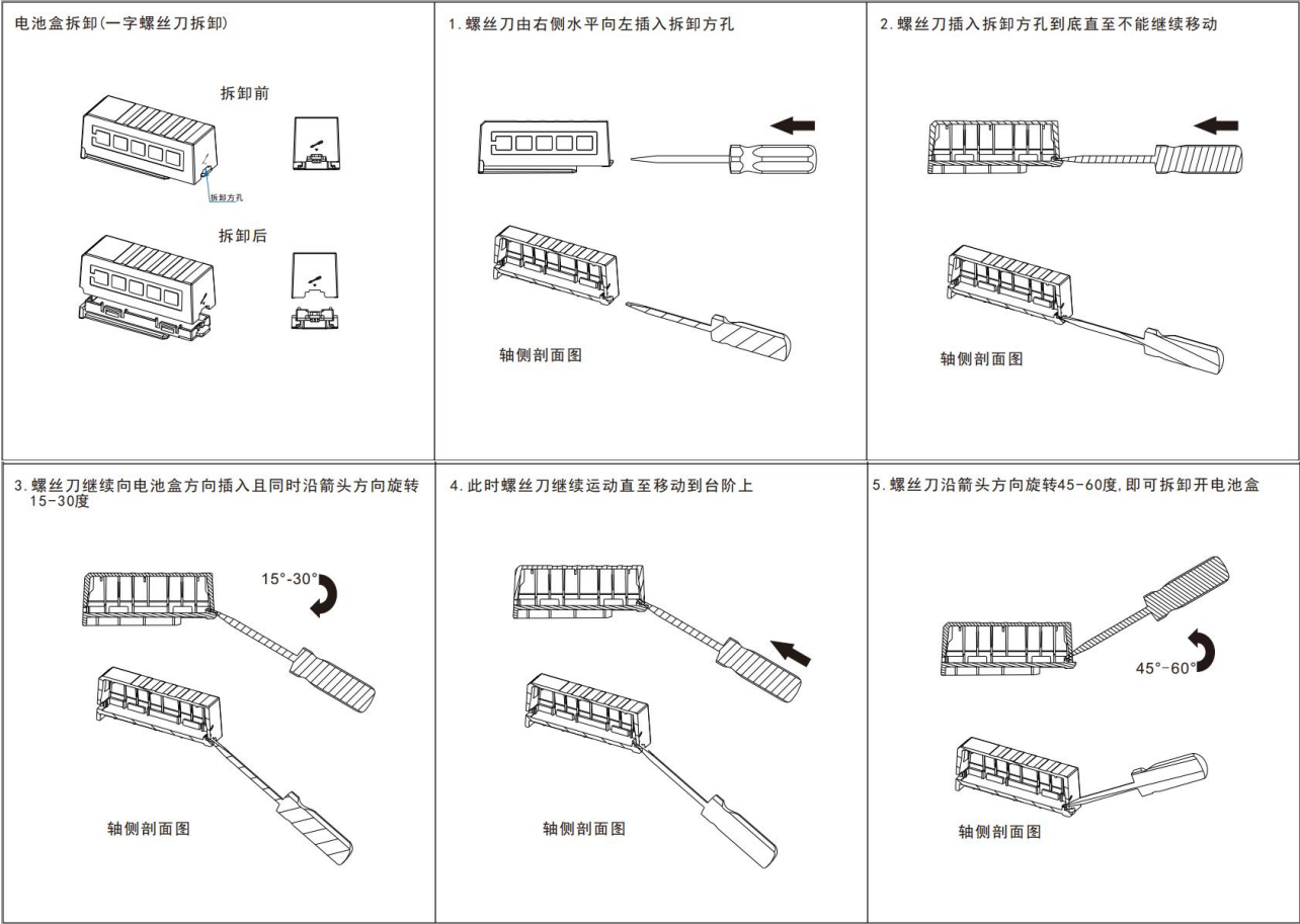
图 6-19 电池盒拆卸方式
