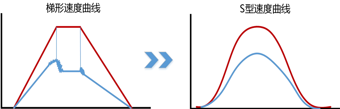
图 7-7 S 型速度阶跃曲线
