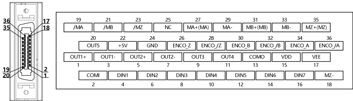
图 3-17 FD5-LA/CA 驱动器外部输入输出端子引脚示意
