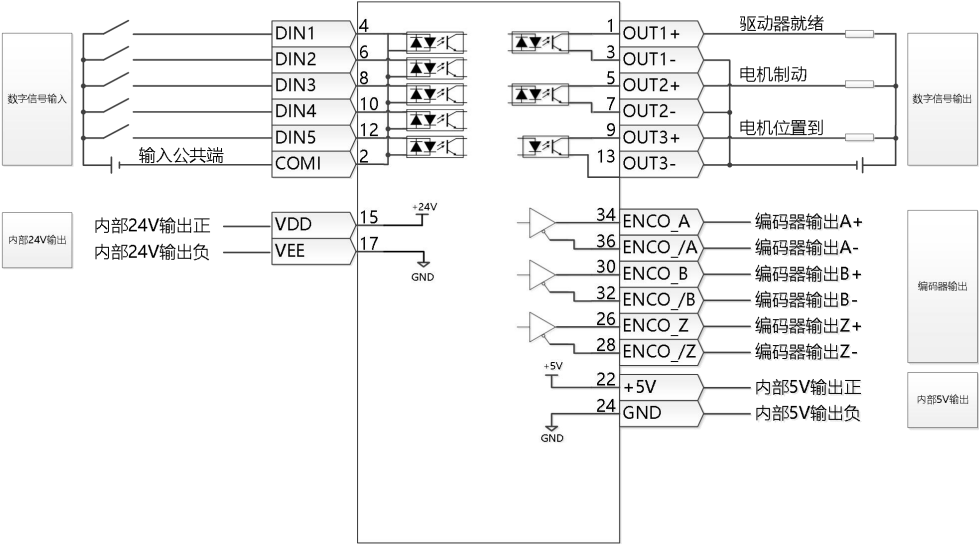
图 3-20 FD5-PA 驱动器 IO 口默认定义
