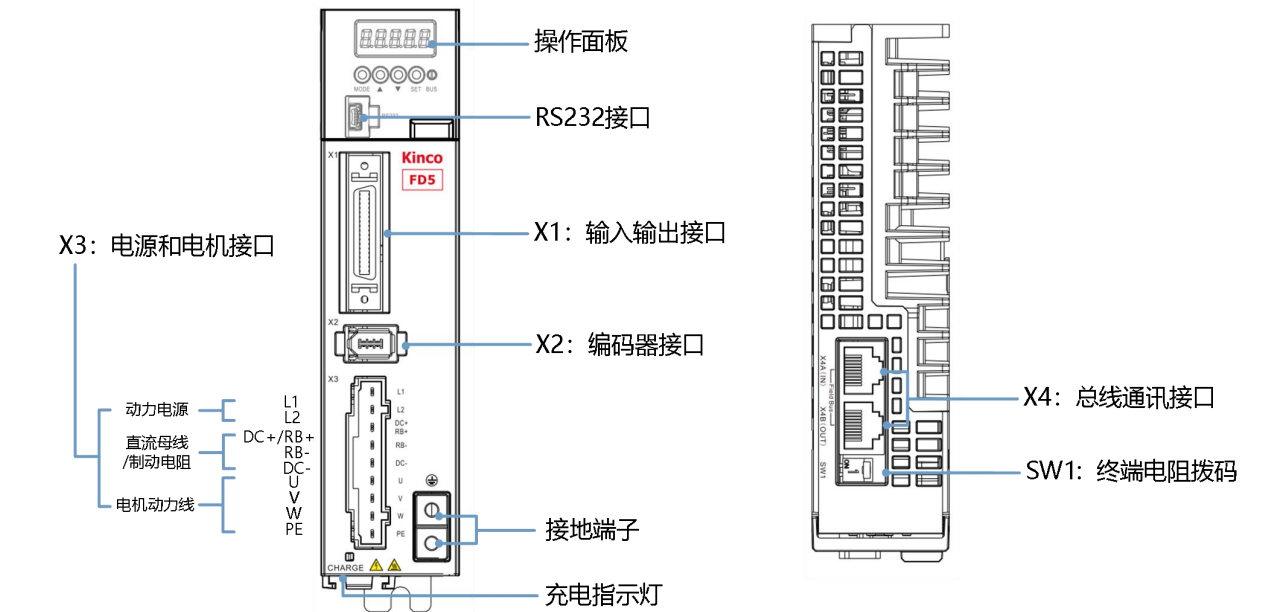
图 3-1 FD425 驱动器外观图
