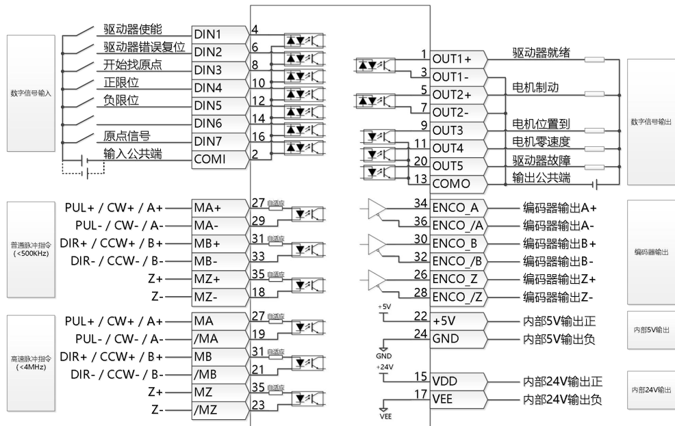
图 3-18 FD5-LA/CA 驱动器 IO 口默认定义
