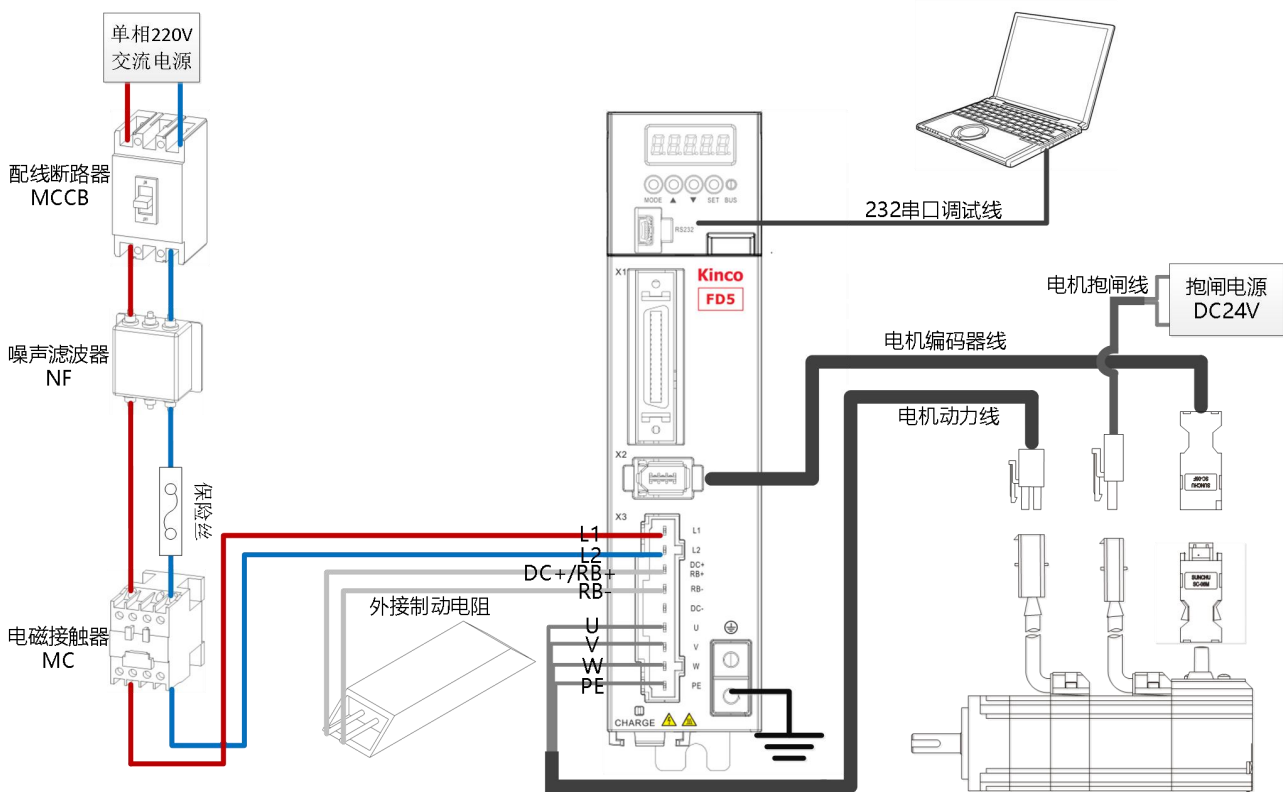
图 3-3 FD425 外部接线图
