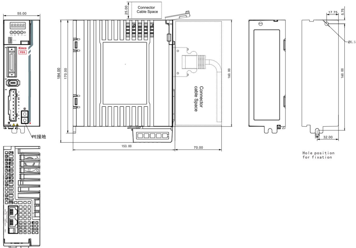
图 2-2 FD425-□F 产品安装图
