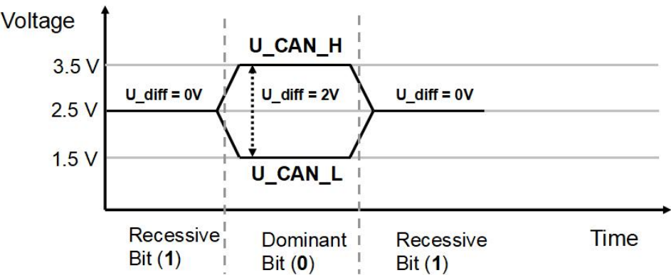
图 10-3CAN 信号标识
