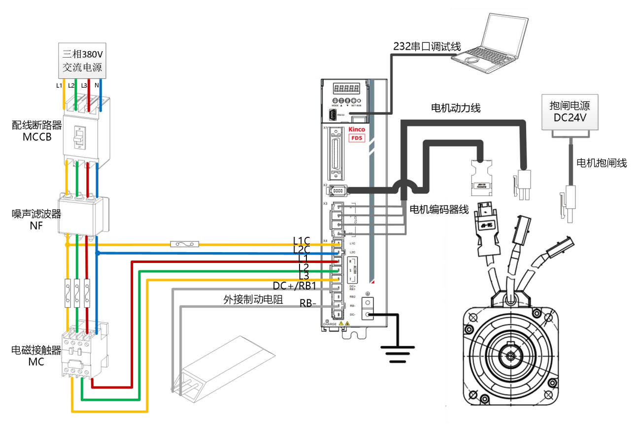
图 3-5 FD625 外部接线图
