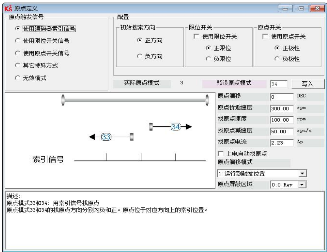
图 6-15 原点定义设置界面
