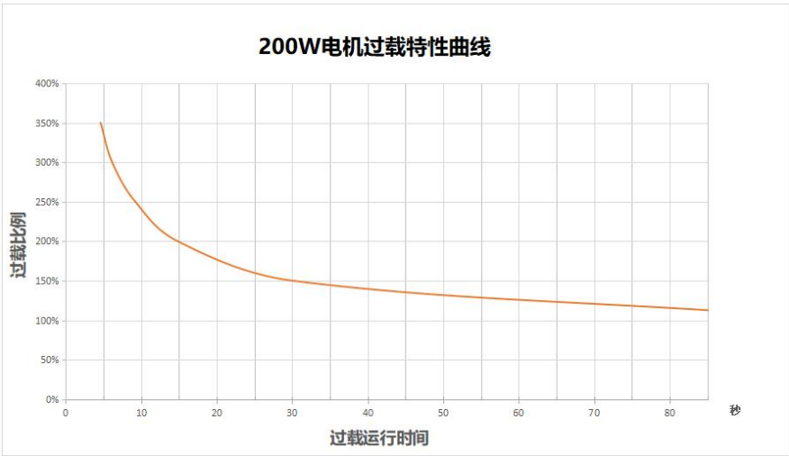
图 3-11 200W 电机过载特性曲线
