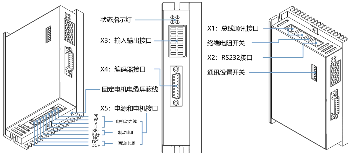
图 3-1 FD123 驱动器各部分名称
