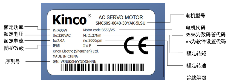
图 1-2 电机铭牌
