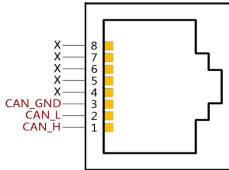
图 5.4-02: CANopen 通讯引脚定义 (RJ45)
