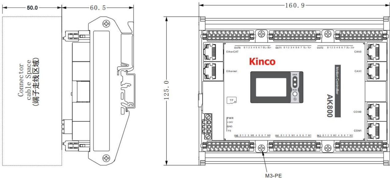
图 3.9-01: AK800 系列控制器外观尺寸示意图 (mm)
