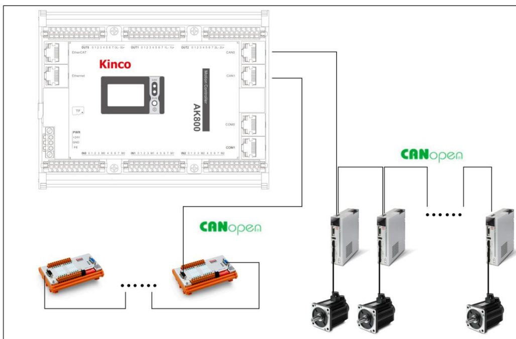
图 5.4-01: CANopen 组网示例
