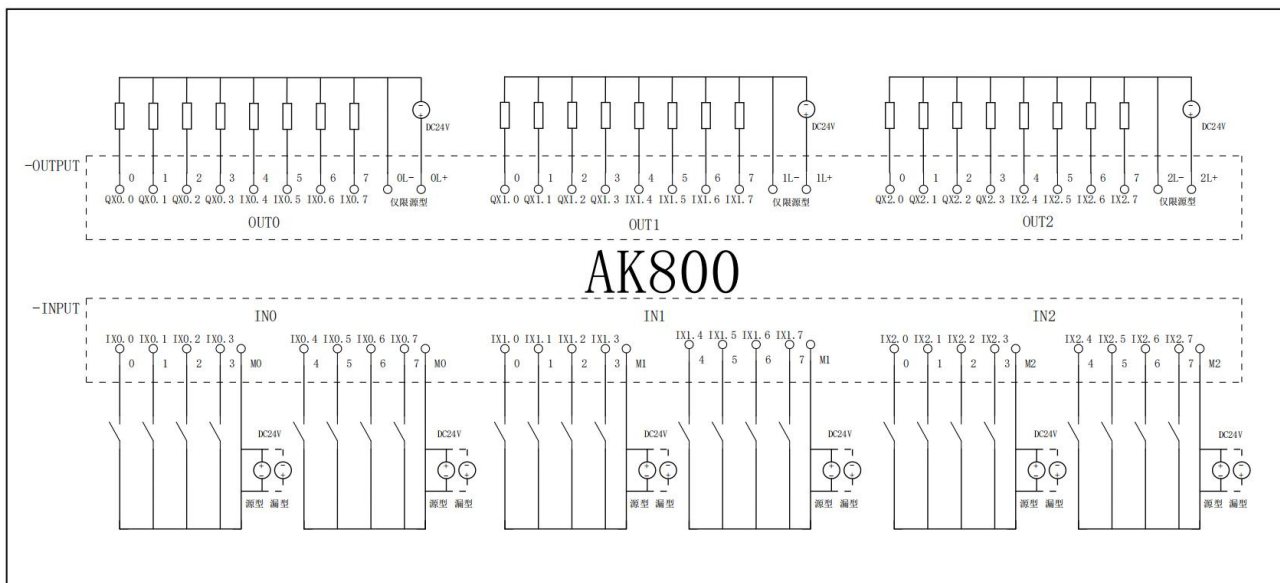
图 5.3-01: AK800 I/O 接线图
