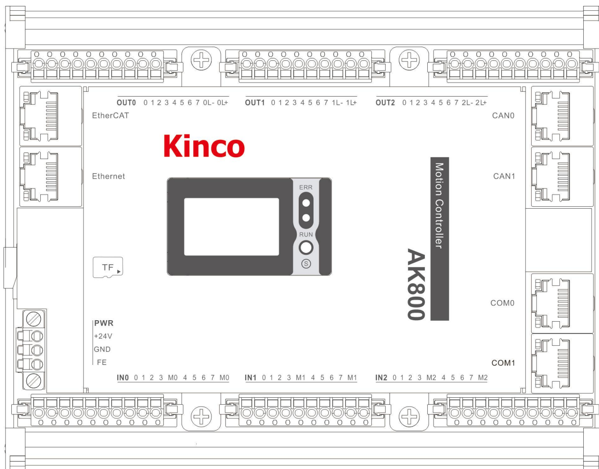
图 2.1-01: AK800 平面图
