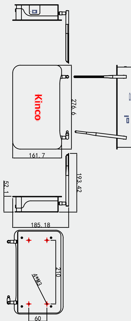
产品尺寸图 (单位: mm)
