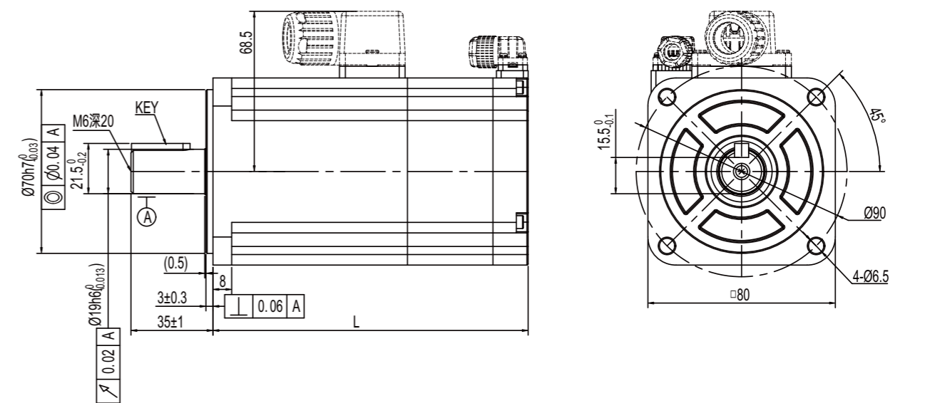
80法兰 (带抱闸)
