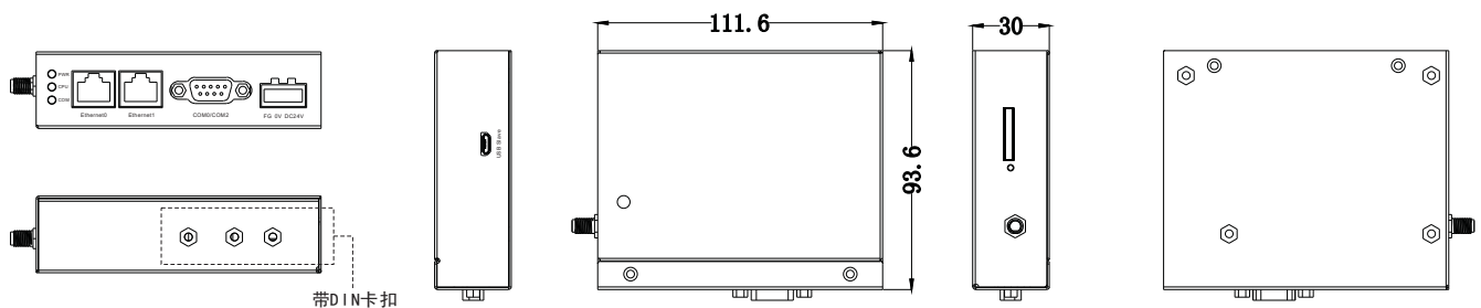
尺寸图: (mm)
