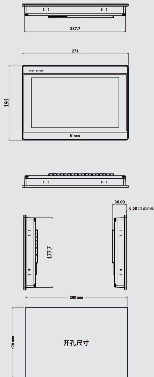
尺寸图(单位:mm)
